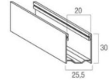
Guida in alluminio A27 GUIAL...27M 25,5 x 30 mm
