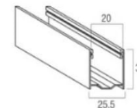
Guida in alluminio A27 GUAL...27M 25,5 x 30 mm
